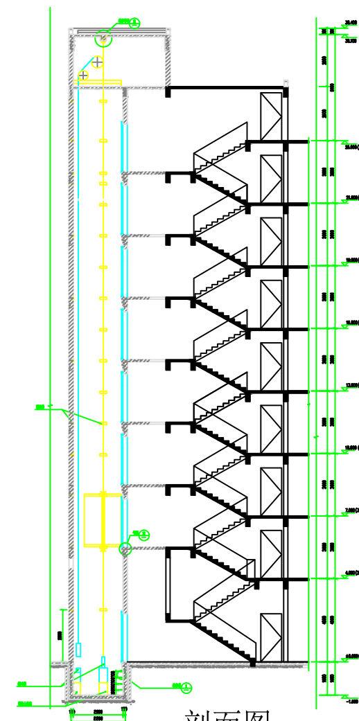
剖面图
